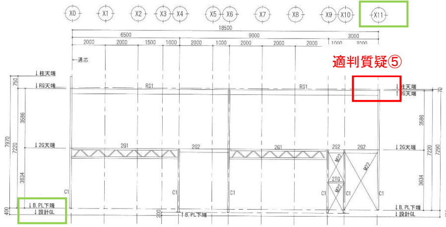
通り軸組図
