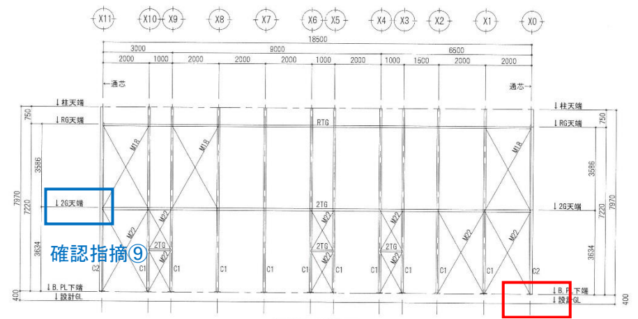
通り軸組図
