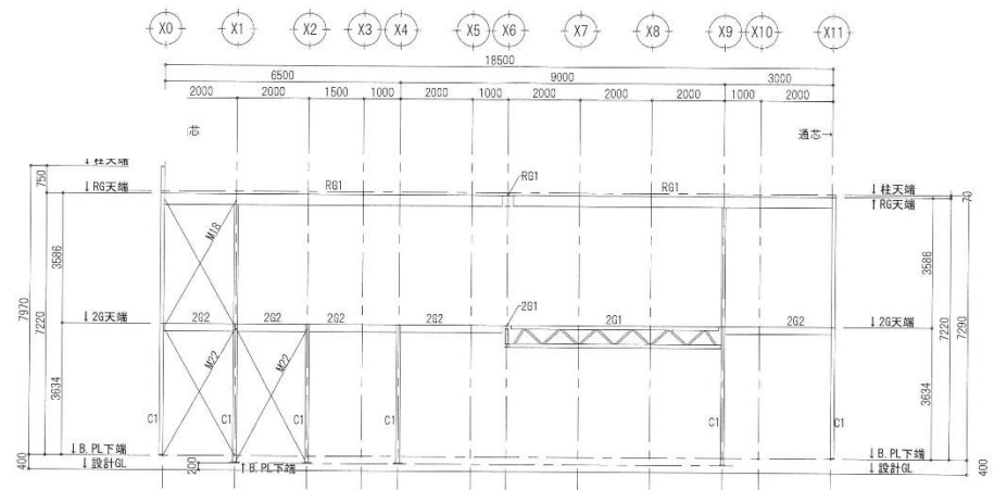
通り軸組図
